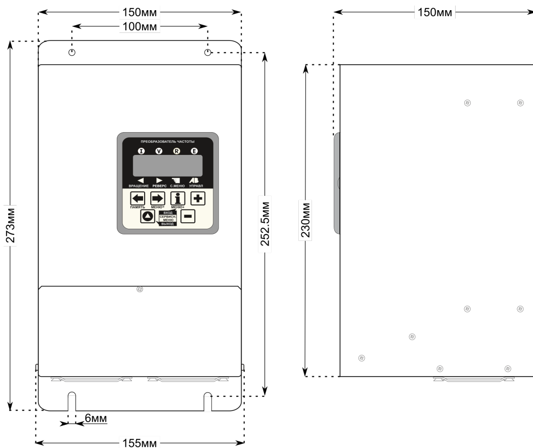
Рисунок 1в. Габаритні розміри перетворювачів CFM310 4.0кВт, 5.5кВт, 7.5кВт, 11кВт.
