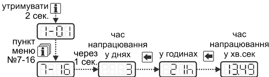
Рисунок 28. Приклад відображення часу напрацювання.
