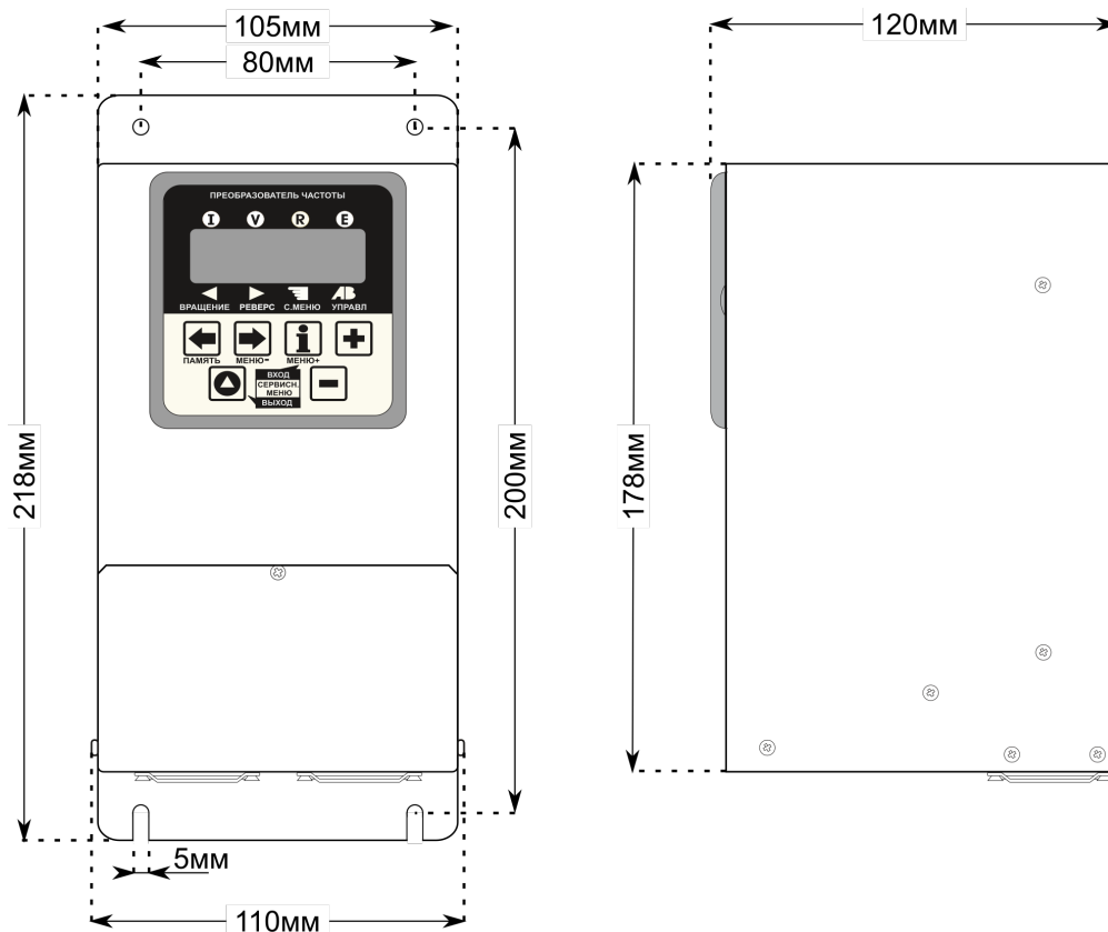
Рисунок 1а. Габаритні розміри перетворювачів CFM310 1.1 та 1.5кВт.
