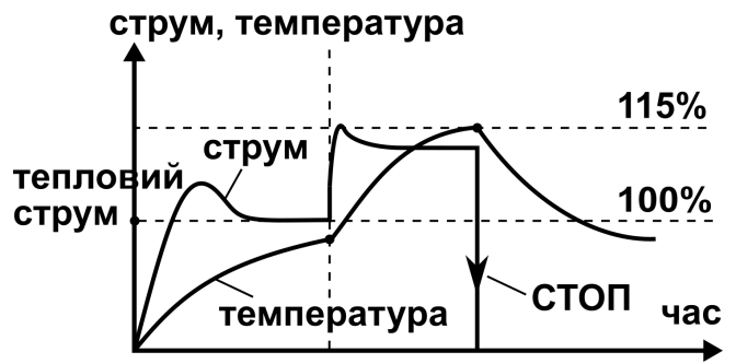
Рисунок 23. б) Принцип дії захисту по перегріву двигуна.
