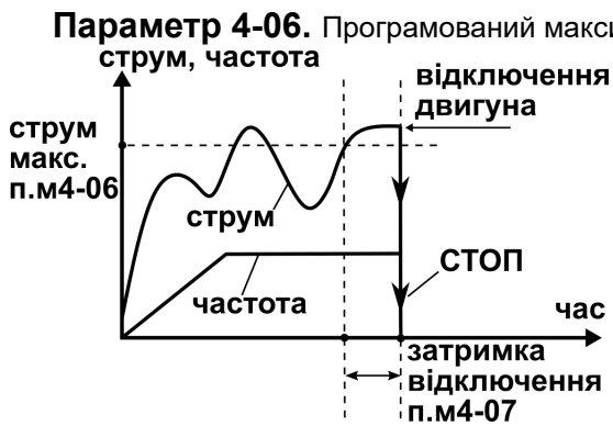
Рисунок 16. Принцип роботи програмованого захисту по максимальному струму двигуна.
