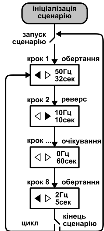
Рисунок 27. Приклад виконання програмованого сценарію.
